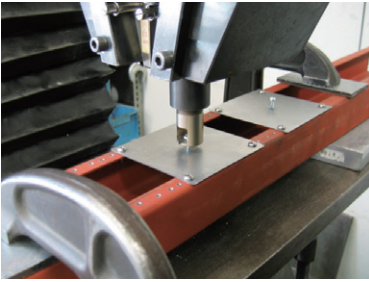
鋼製下地への留め付け方法確認試験
