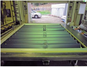
折板軒出長さ耐力試験
