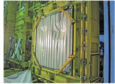
飛来物耐衝撃性能試験
