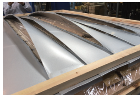
一文字ぶきの耐風圧性試験
