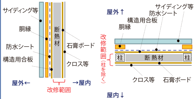
図2-1 横から見た断面図
