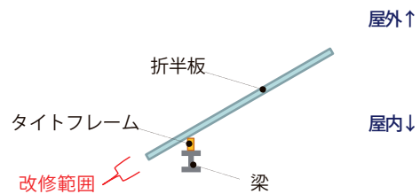
図3 横から見た断面図
