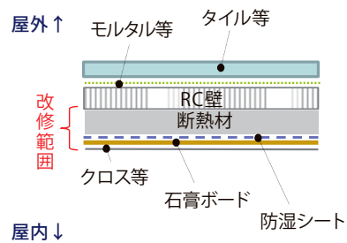
図2-6 上から見た断面図
