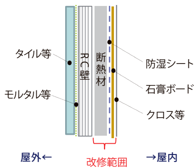
図2-5 横から見た断面図
