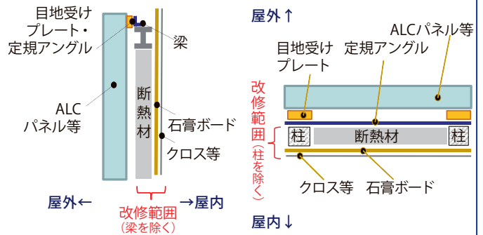
図2-3 横から見た断面図
