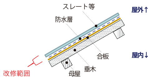
図1 横から見た断面図
