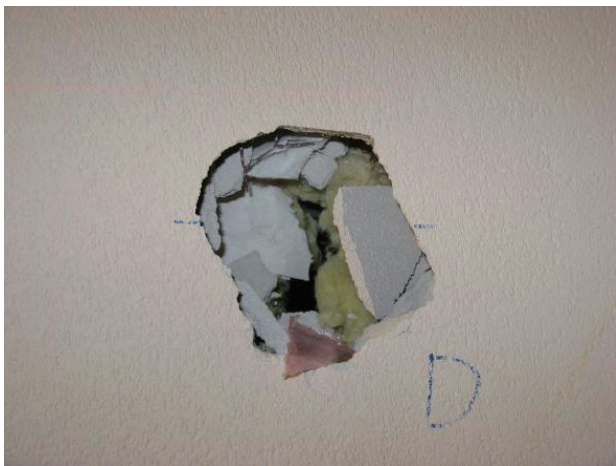
(17) 試験体No.6、ミサイルDの貫通痕
