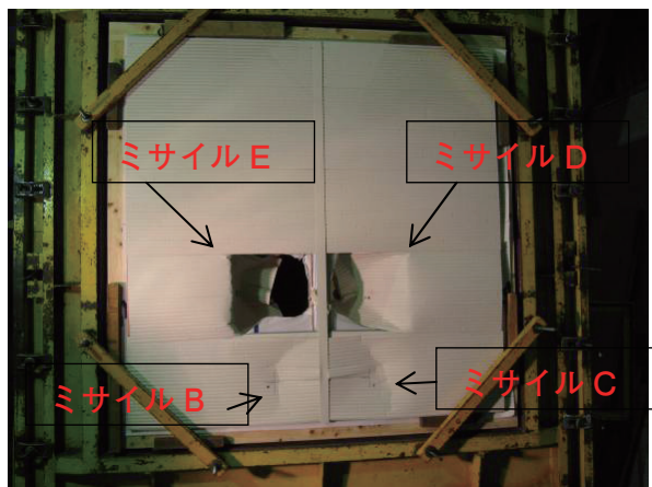
(7) 試験体No.3
