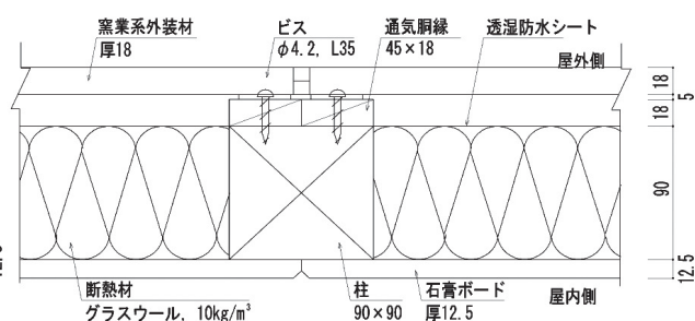
(2) 試験体No.2 (窯業系サイディング厚さ18mm)
