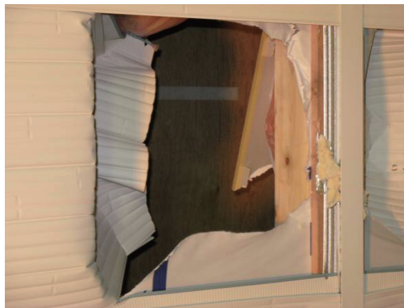
(8) 試験体No.3のミサイルEによる貫通
