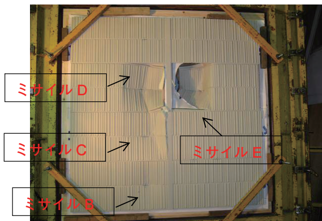
(9) 試験体No.4
