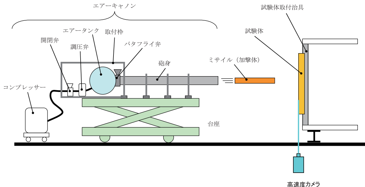
図2 飛来物耐衝撃試験装置概略図
