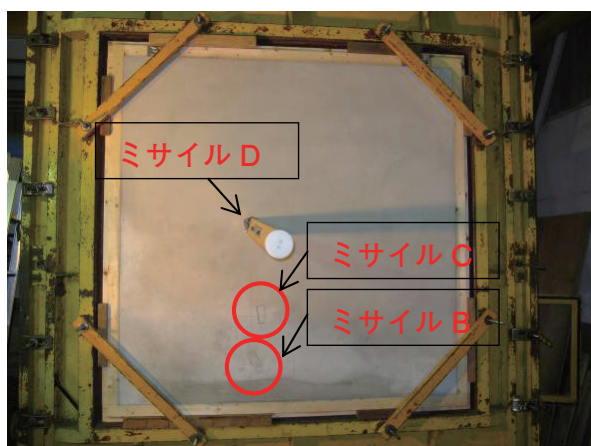
(11) 試験体No.5、ミサイルDの突き刺さり
