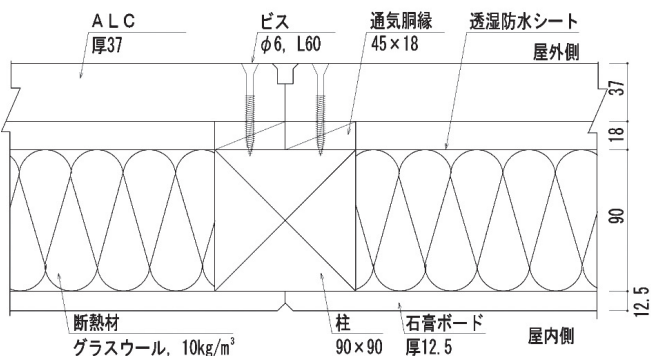
(6) 試験体No.6 ALCパネル
