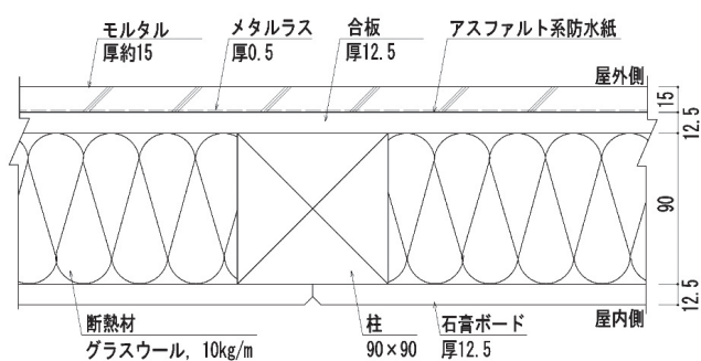
(5) 試験体No.5 (ラスモルタル塗壁)
