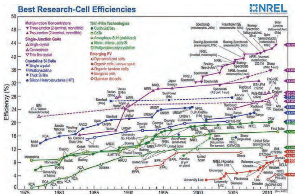
図2-1 太陽光パネル効率変遷
