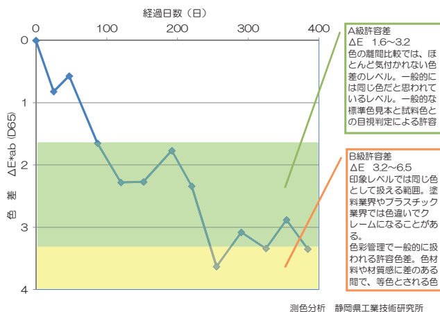
図8-2 褪色測色分析
