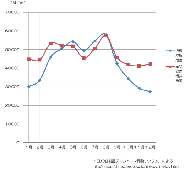
図3-3 折板屋根と年間最適傾斜角比較 (浜松市、方位角340度)
